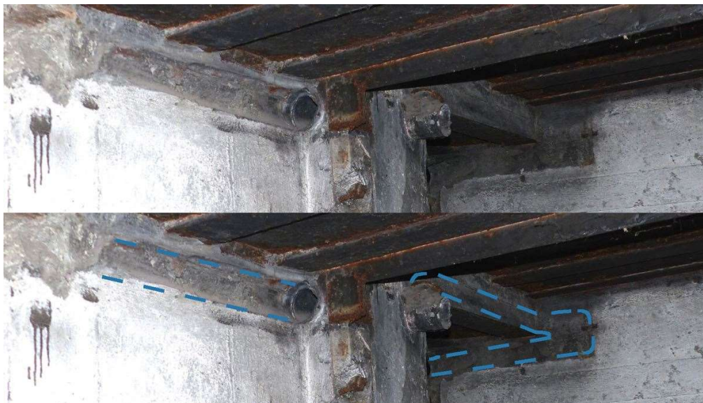
Fot. 13. Wyjątkowo ciekawa pozostałość po przewodzie wyrzutu gazów prochowych. Widoczny fragment przechodził z korytarza (e) przez śluzę pgaz (h) do izby bojowej (g). Przerwaną linię oznaczono próbę rekonstrukcji przebiegu rury.
