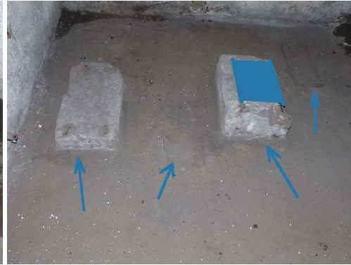
Fot. 05. Maszynownia. Od lewej: żelbetowa podstawa wentylatora ręcznego, ślad mocowania prądnicy, żelbetowa podstawa silnika (częściowo uszkodzona), ślad mocowania wentylatora mechanicznego. Na podstawie silnika zaznaczono niebieskim konturem sylwetkę spodu silnika Blackstone DB 3. Stan na luty 2021.
