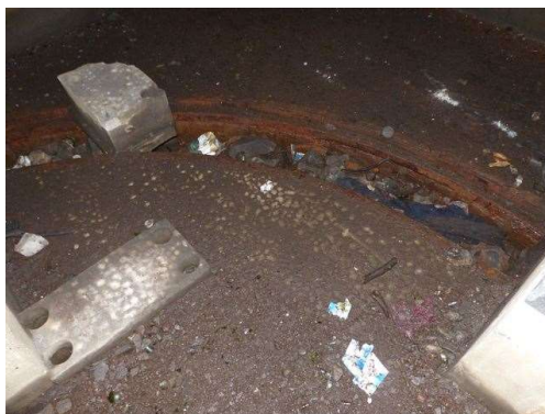
Fot. 10. Maszynownia nieukończonego schronu nr 42a. Po lewej stronie podstawa wentylatora ręcznego, nieco powyżej podstawa silnika. Zwracają uwagę otwory technologiczne na osadzenie szpilek. W centrum kadru kanał podłogowy ze stalowym wzmocnieniem krawędzi. Fot. Łukasz Drzensła.
