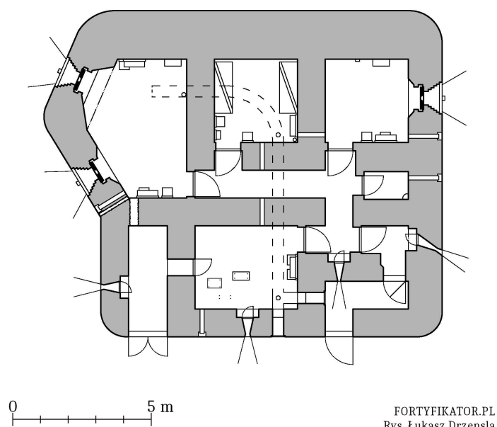
Rys. 01. Plan schronu.
