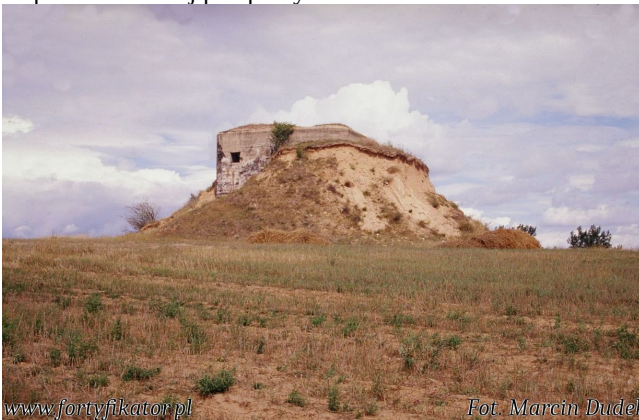
Fot. 12. Schron dowodzenia Darewo 24. Pagórek, na którym zbudowano obiekt został po 2 wojnie światowejNa kopule widoczne zachowane jeszcze ślady farby rozkopany kopany aby powiększyć i zniwelować okolicznemaskowania. Kolor mocno rozbielonego różu może być kołchozowe pole. Widoczny otwór po lewej stronie to efektem płowienia. Jednak można go spotkać praktycznie na wszystkich zachowanych kopułach tego typu.
